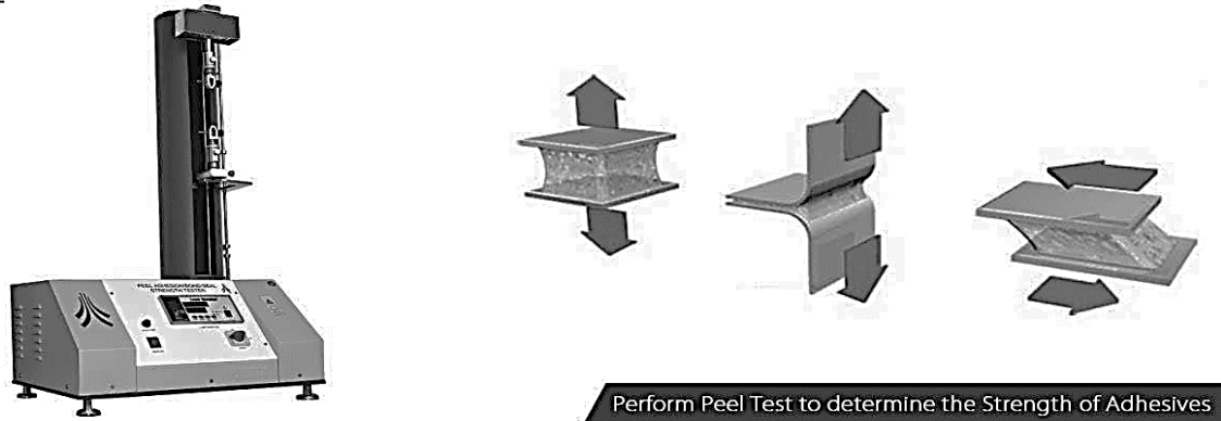
Fig.10.3. Peel Tester
